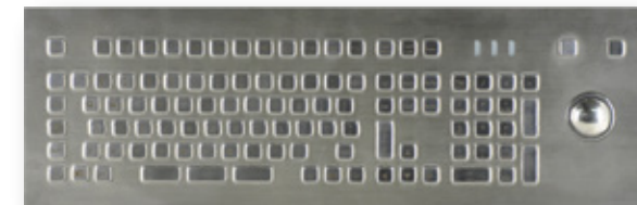
W103T-P TASTIERA IN ACCIAIO INOX 103 TASTI DA PANNELLO CON TRACKBALL
